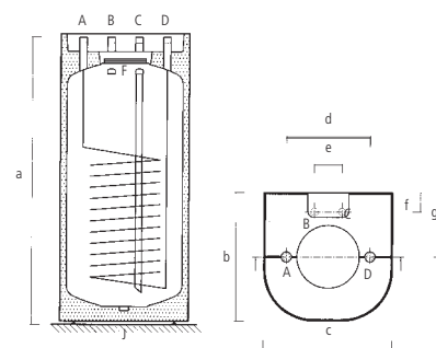
Type 2440, 2443 110 liter med kabinet
