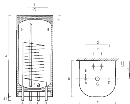
Type 6220, 2623, 6440, 2643, 6050, 2653 60-110-160 liter med kabinet
