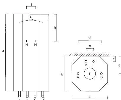
Type 6441 110-150 liter uden kabinet
